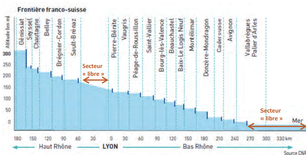
Figure 18 : Répartition des aménagements sur le Rhône français (source : le Rhône en 100 questions)
