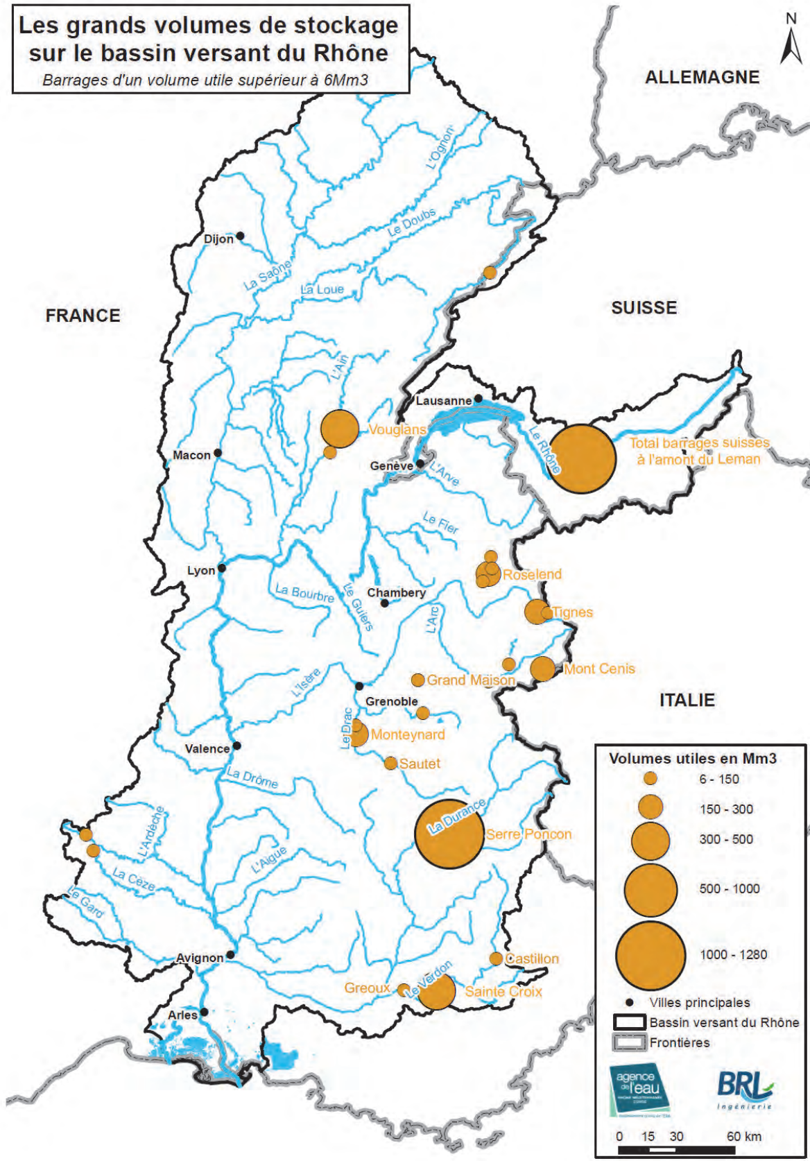
Figure 6 : Ouvrages de stockage
