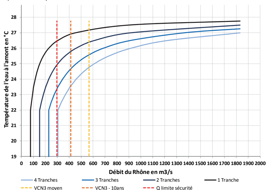
Figure 52 : Conditions limites en débit et température pour le fonctionnement des tranches ouvertes de la centrale de Tricastin (source : EDF)
