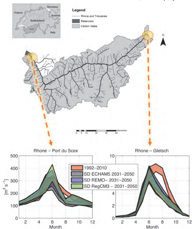
Figure 54 : Simulations des débits du Rhône à Gletsch et Porte du Scex, dans le projet ACQWA 5
