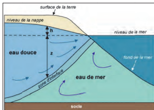
Figure 30 : Schématisation d'un biseau salé dans un aquifère homogène.
