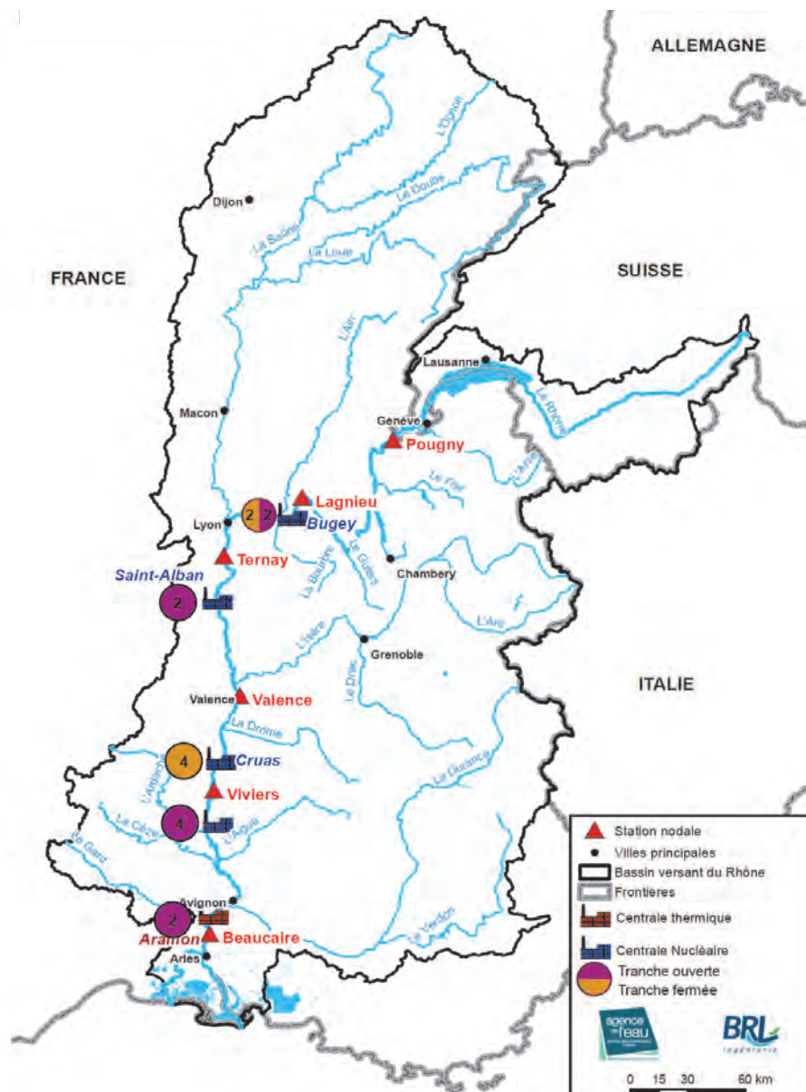
Figure 34 : Les centrales nucléaires et thermique de production d'énergie sur le Rhône
